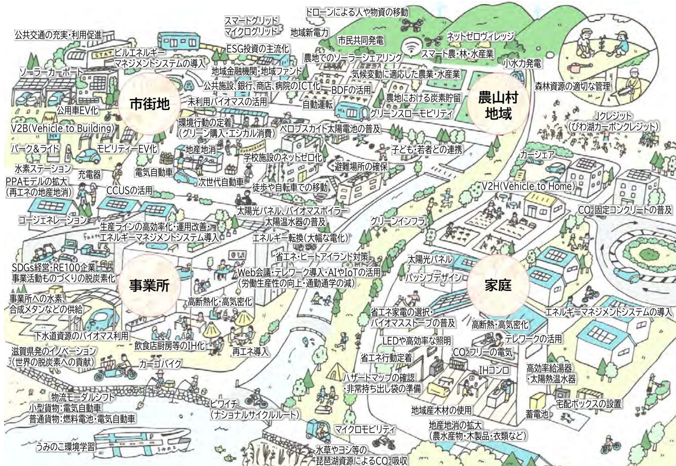
図6 2050年CO 2 ネットゼロを達成した滋賀県の姿
